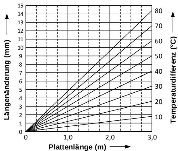
Diagramm über die Ausdehnung von VEKAPLAN S / SF / CX-DUO-Platten
