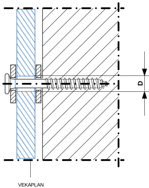
direkte Verschraubung
