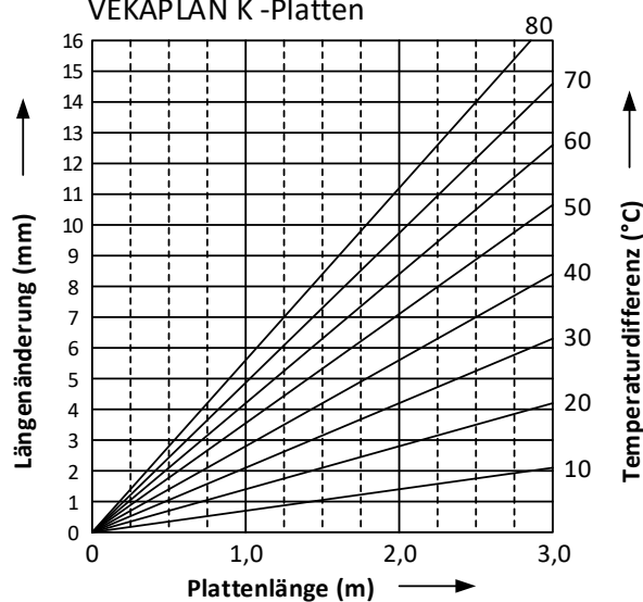
Diagramm über die Ausdehnung von VEKAPLAN K -Platten
