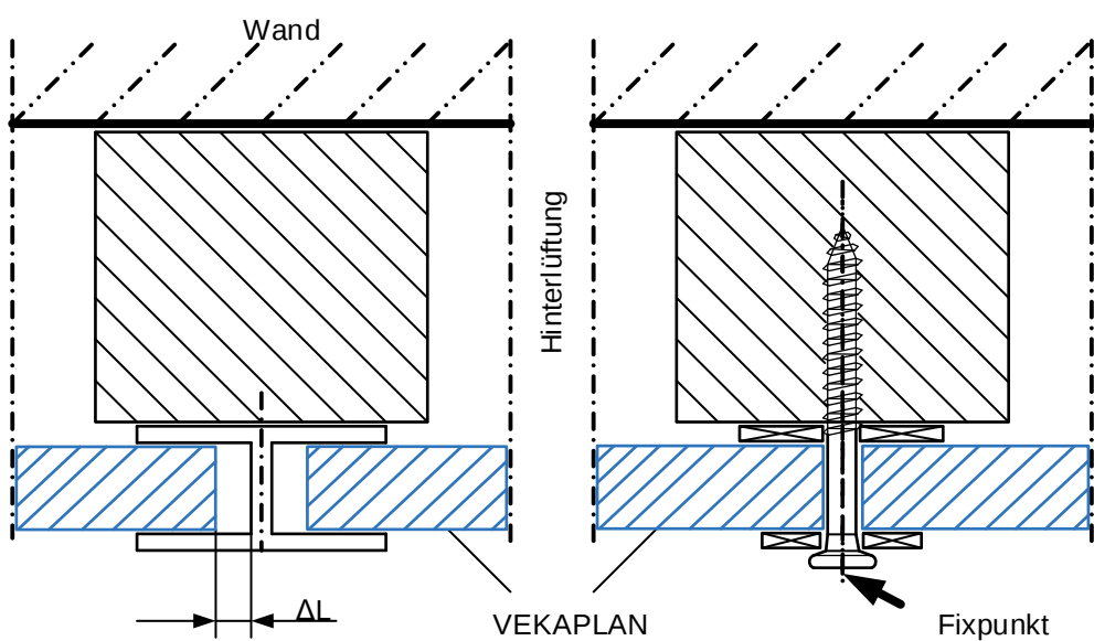
Montage, hinterlüftet
